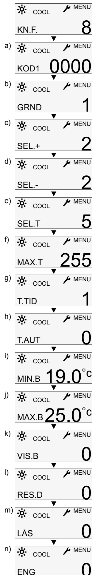
Menyn för knappfunktioner
