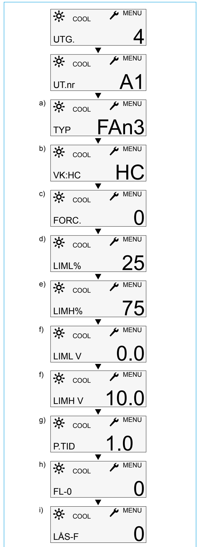
Utgångsmenyn, utgång A1 för fläkthastighetsstyrning
