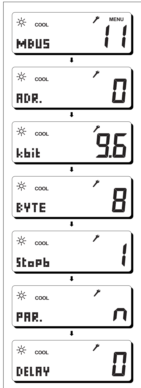
kommunikationsmenyn
